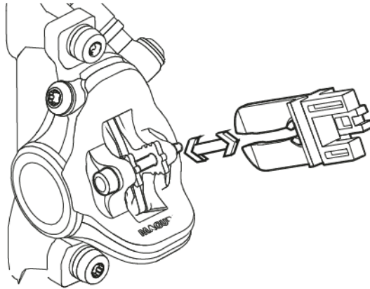
Abbildung 17: Transportsicherung befestigen
