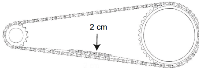
Abbildung 53: Ketten- bzw. Riemen ­ spannung prüfen
