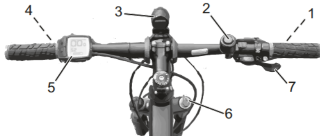
Abbildung 3: Detailansicht Fahrrad -aus Fahrerposition, Beispiel nuclar
