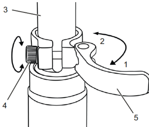
Abbildung 36: Schnellspanner der Sattelstütze (3) mit Spannhebel (5) und Einstellschraube (4) in geöffneter Position (1) und die Richtung der geschlossenen Position (2)
