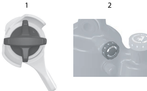
Abbildung 94: Zugstufeneinsteller Float DPS (1) und Float X (2)
