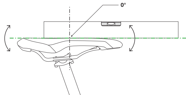
Abbildung 72: Waagerechte Sattelneigung mit 0° Neigung in der Sattelmittle
