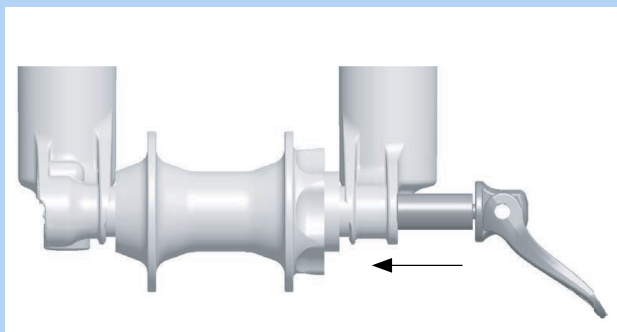
Abbildung 55: Schnellspanner einschieben
