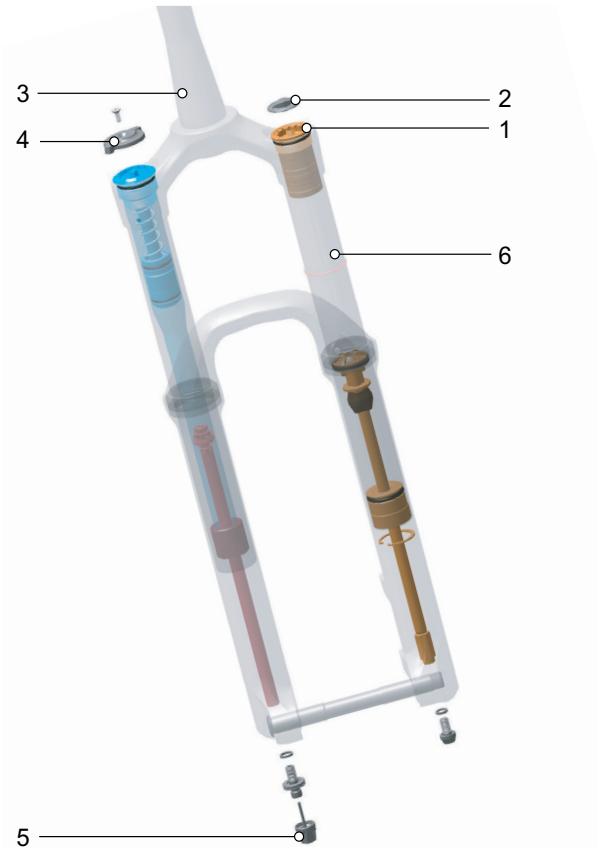
Abbildung 15: Innerer Aufbau Luftfedergabel
