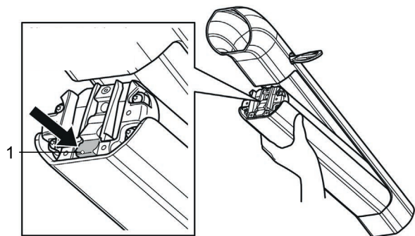
Abbildung 122: Zweifach-Verschlussplatte (1)
