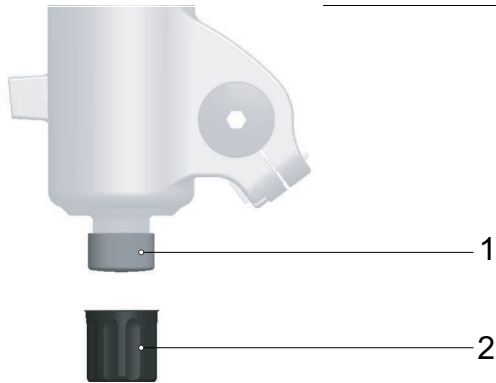
Abbildung 92: FOX Zugstufen-Schraube (1) unter Gabel-Kappe (2)
