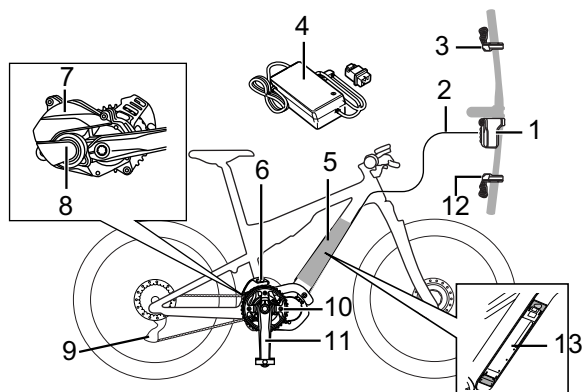
Abbildung 35: Schema Elektrisches Antriebssystem
