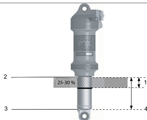
Abbildung 90: (1) SAG, Gummi-Luftkammer-Dichtung (2), O-Ring und Gesamtfederweg des Dämpfers
