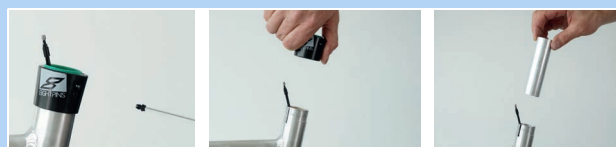
Abbildung 201: Außenhülle und Gleitbuchse ausbauen
