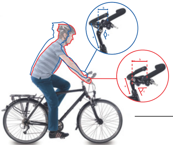
Figura 80: Posición de la bicicleta de ciudad (azul) y la bicicleta de trekking (rojo) mediante la modificación angular
