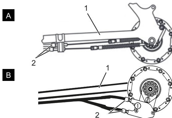
Figura 154: Casquillos de ajuste (2) en dos versiones alternativas (A y B) de un cambio de marchas accionado por cable de accionamiento, de dos cables en la vaina (1)
