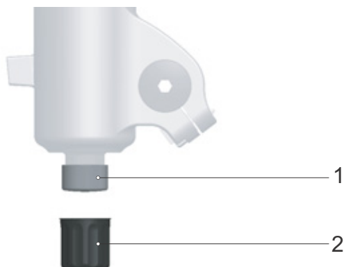
Figura 222: Tornillo de niveles de tracción FOX (1) debajo del capuchón de la horquilla (2)
