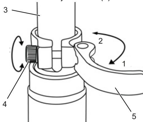
Figura 68: Apertura del cierre rápido de la tija de sillín
