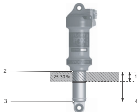
Figura 90: (1) SAG, junta de goma de la cámara de aire (2), junta tórica y recorrido de muelle total del amortiguador
