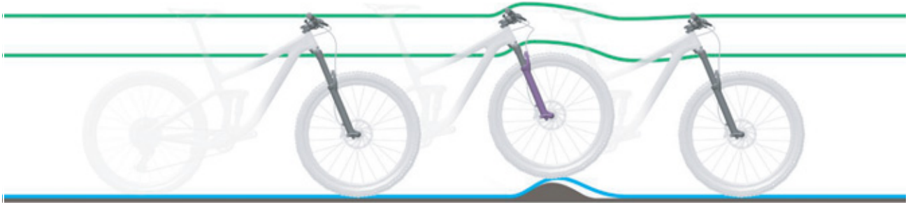
Figura 228: Amortiguación de la horquilla de suspensión demasiado dura en caso de irregularidades
