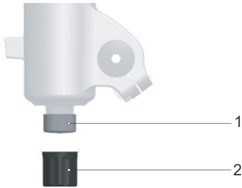
Figura 92: Tornillo de niveles de tracción FOX (1) debajo del capuchón de la horquilla (2)
