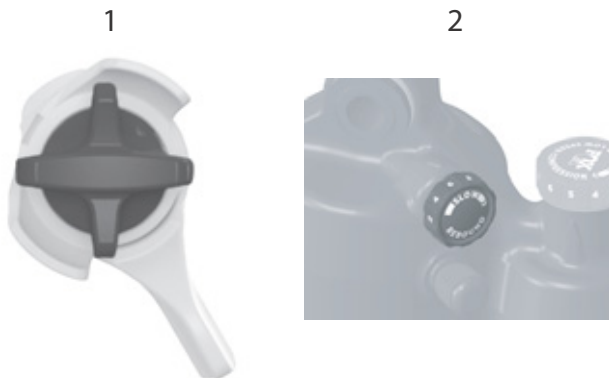
Figura 232: Regulador de niveles de tracción Float DPS (1) y Float X (2)
