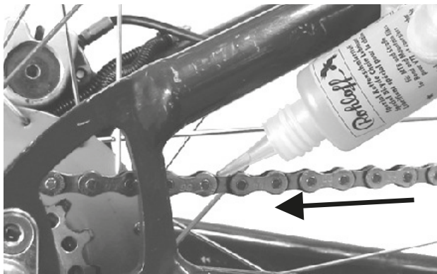
Figura 143: Lubricación de la cadena
