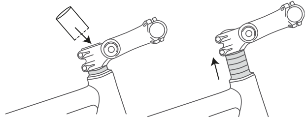
Figura 78: Aumento de la potencia Ahead mediante el montaje de anillos distanciadores (separadores)
